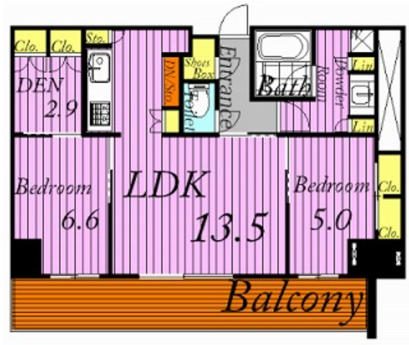
【間取り図】
